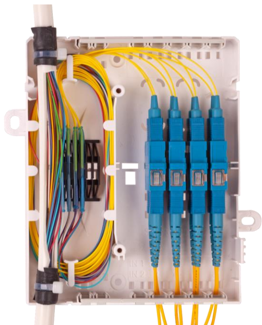
Řešení s Riser kabelem (Ukončení 8 vláken)
