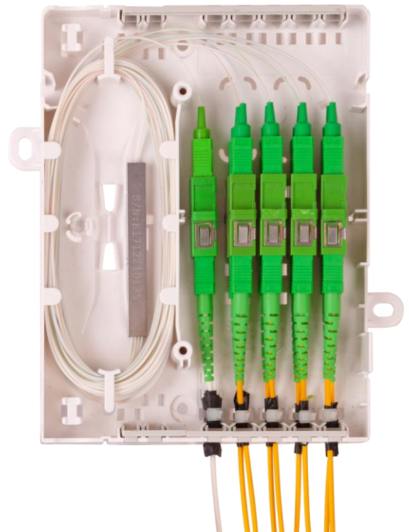
Řešení bez svárů se splitterem 1:8 (levý adaptér vstup splitteru)
