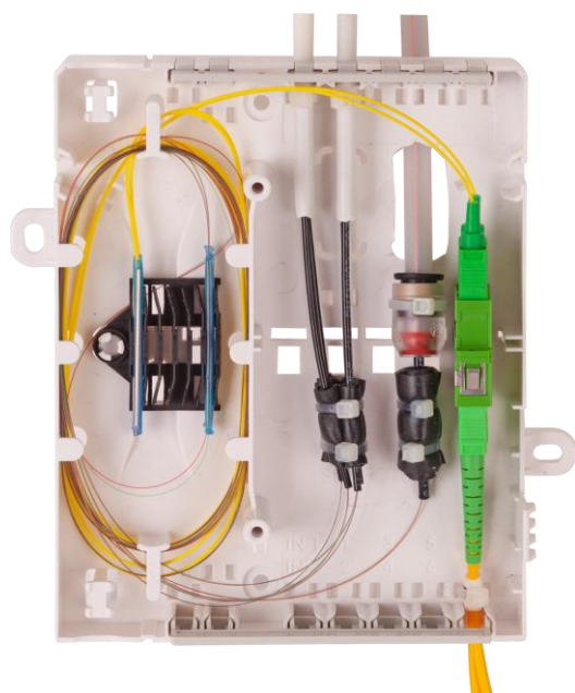
Řešení se vstupem přes stěnu a kombinace připojení zákazníků
