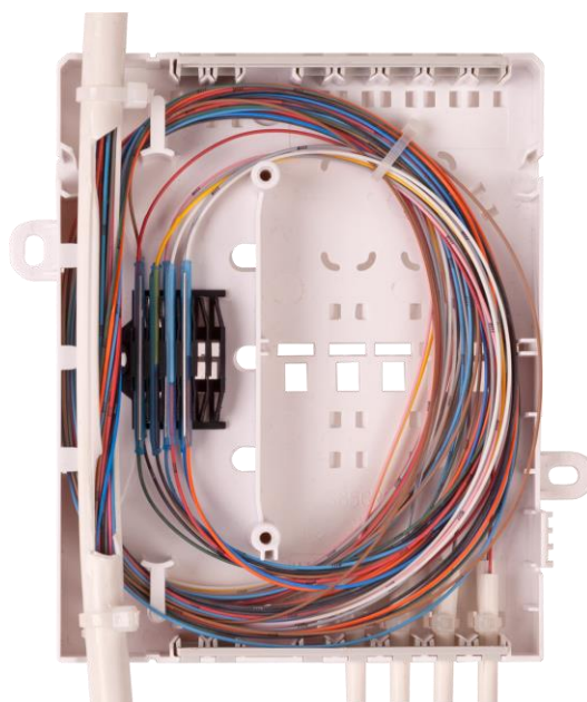
Řešení s Riser kabelem (pouze svařování)
